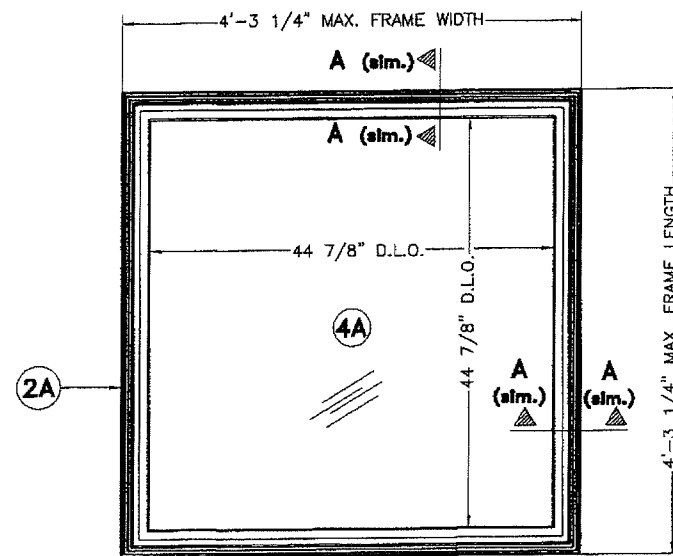
PLAN (INTERIOR SIDE) N.T.S.
