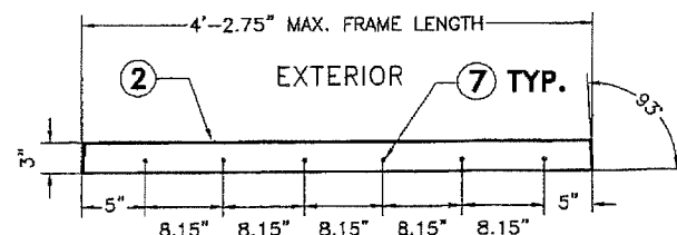
VIEW Y
