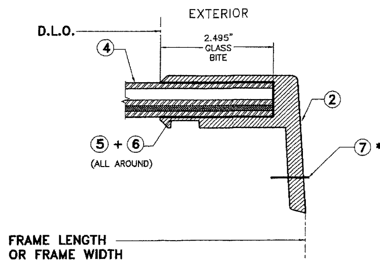
SECTION A-A SCALE: 1/2"=1"
