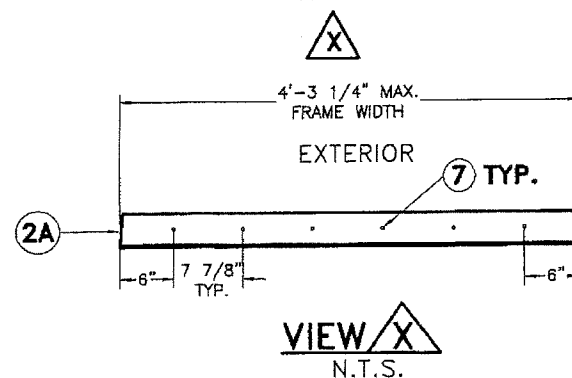
PLAN (EXTERIOR SIDE) N.T.S.
